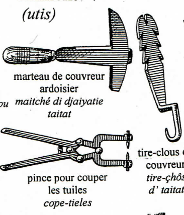
essette de charpentier aïssatte de tchaïpu herminette de charpentier brisadiu d' tchaïpu
